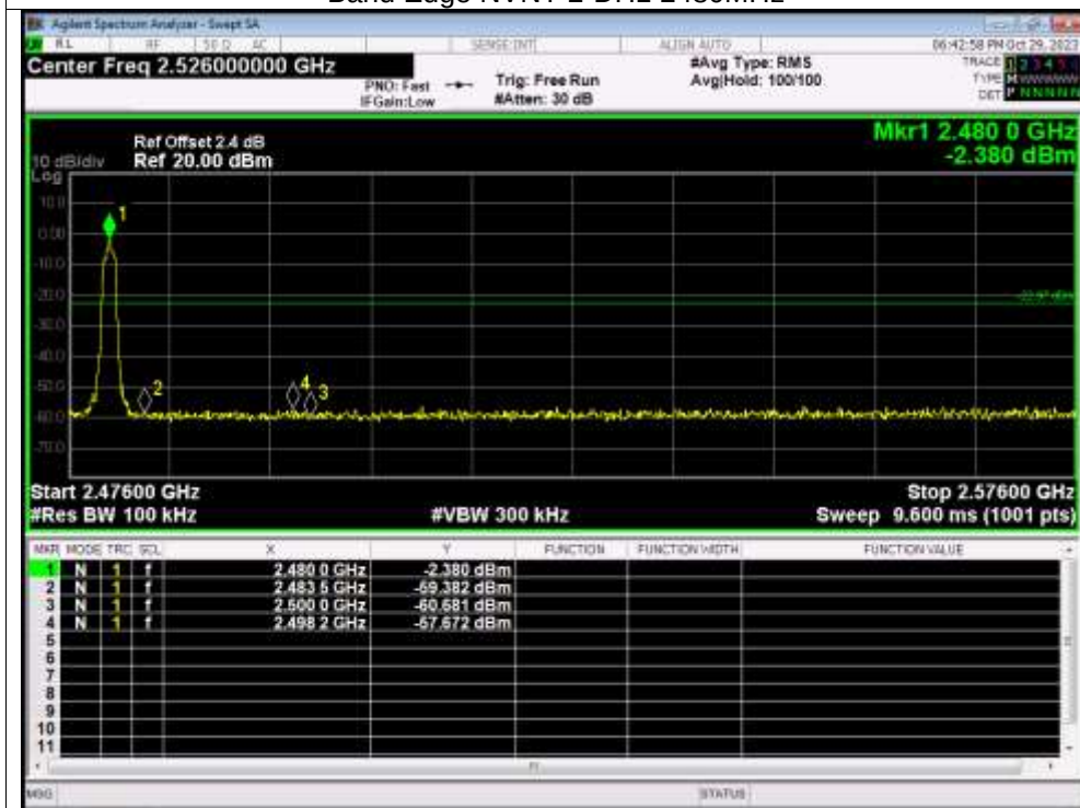
Band Edge NVNT 2-DH1 2480MHz
