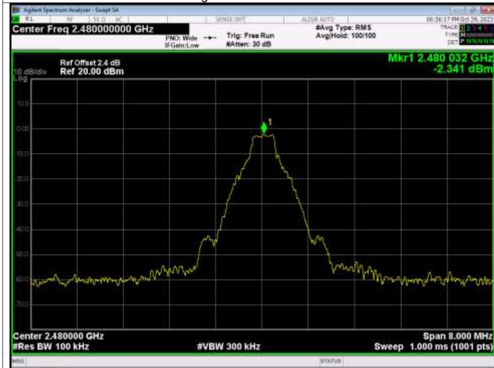
Band Edge NVNT 1-DH1 2480MHz
