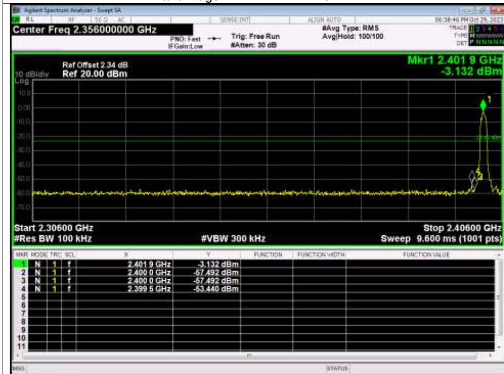
Band Edge NVNT 2-DH1 2402MHz
