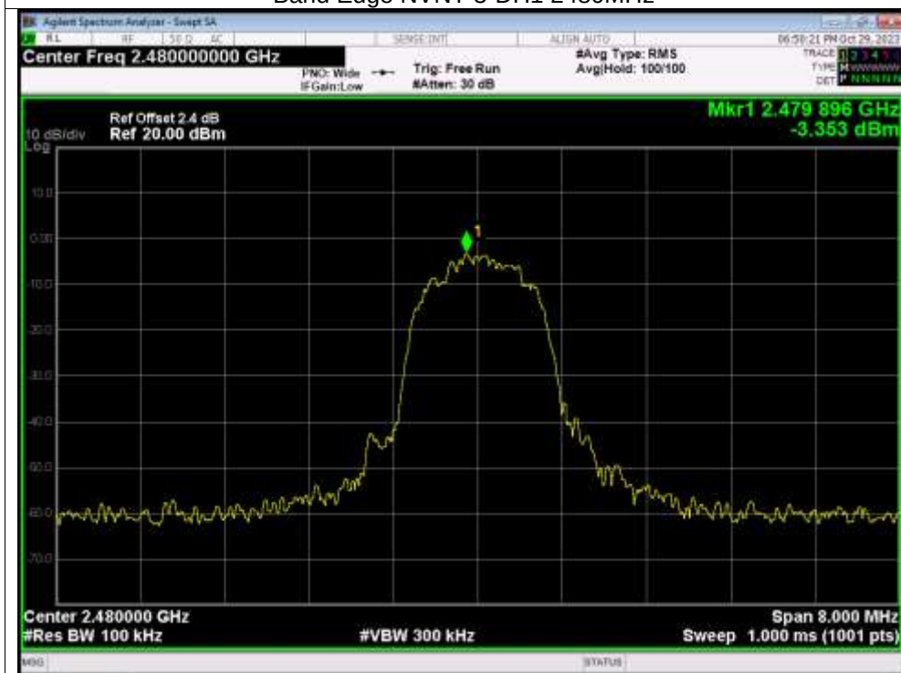
Band Edge NVNT 3-DH1 2480MHz
