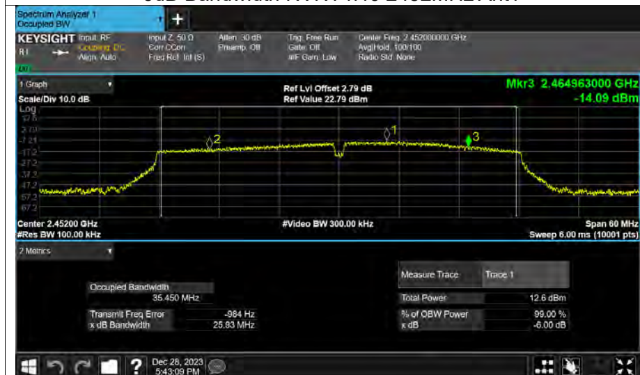
-6dB Bandwidth NVNT n40 2452MHz Ant1
