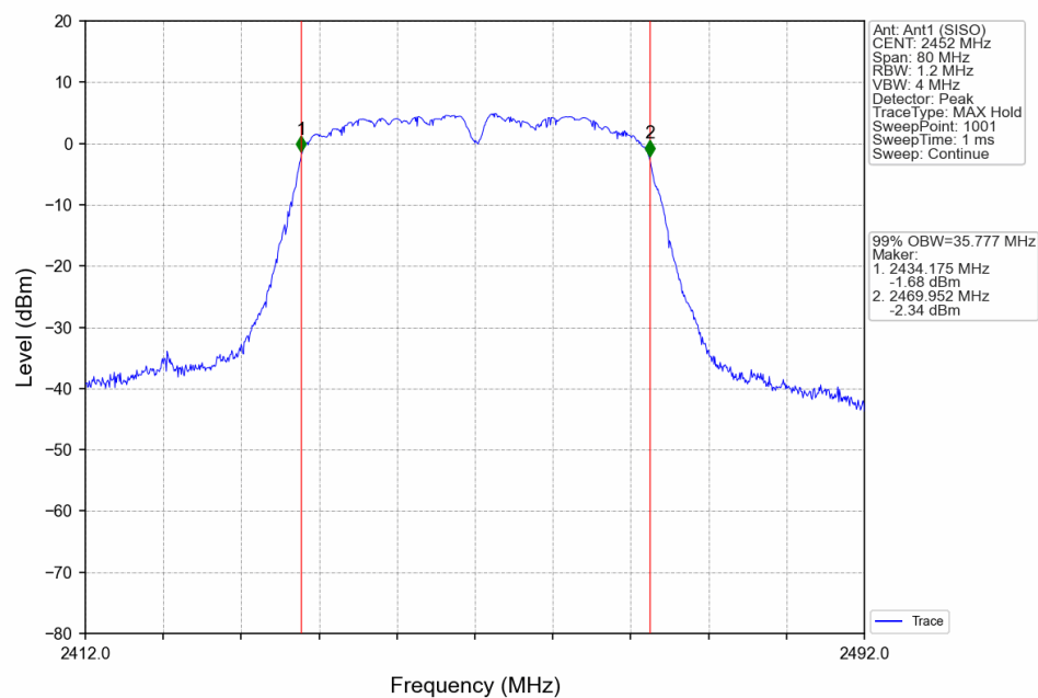
802.11n(HT40) HCH 2452MHz Ant1 (SISO) NTVN
