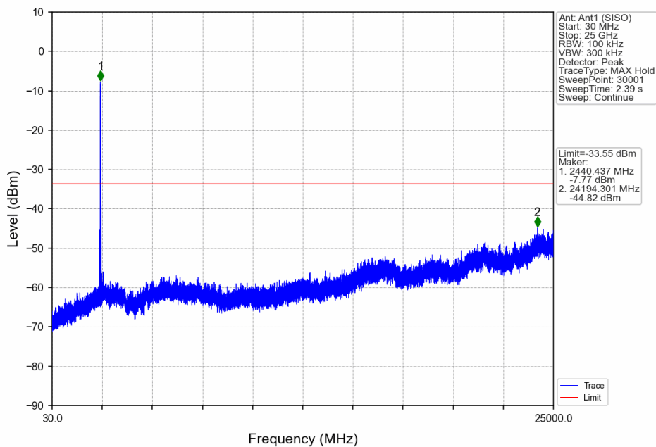
802.11n(HT40) MCH 2437MHz Ant1 (SISO) NTNV
