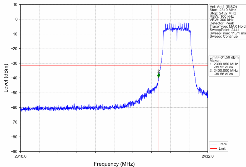
802.11n(HT20) LCH 2412MHz Ant1 (SISO) NTVN
