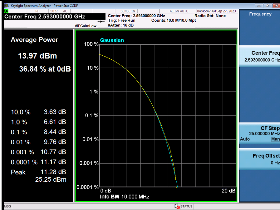
Band41 2593MHz AWGN SISO Ant1 NTVN AGC+3
