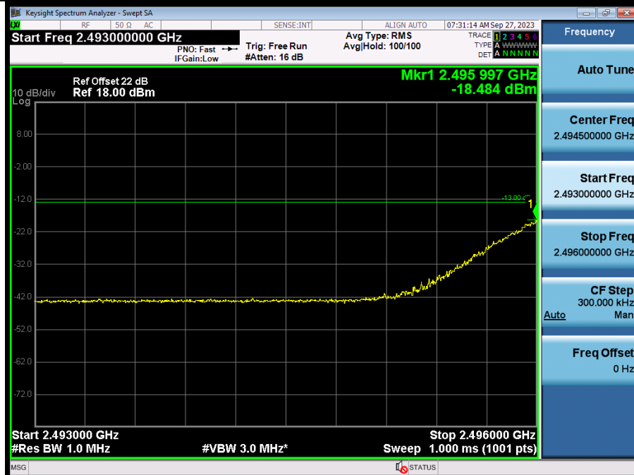
Band41_2546MHz_AWGN_SISO_Ant1_NTNV_AGC+3
