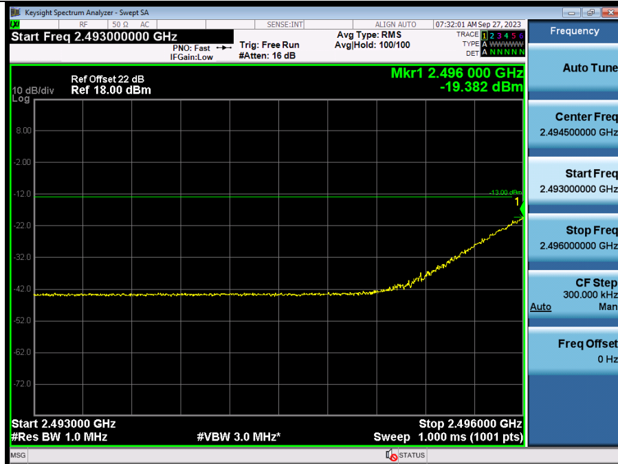
Band41_2546MHz_AWGN_SISO_Ant1_NTNV_AGC+3
