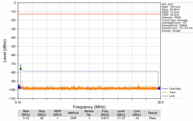
Band41_2593MHz_AWGN_SISO_Ant1_NTNV
