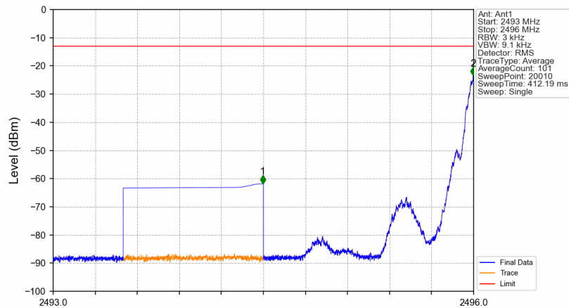
Band41_2496.1MHz_GMSK_SISO_Ant1_NTNV_AGC+3
