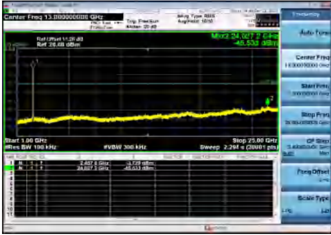
1GHz-25GHz
