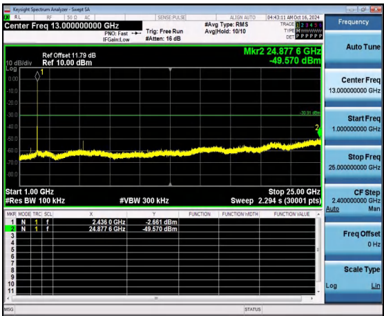
1GHz -25GHz
