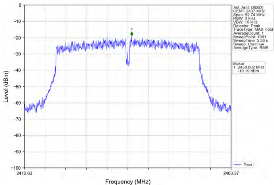
802.11n(HT40)_MCH_2437MHz_Ant4 (SISO)_NTNV
