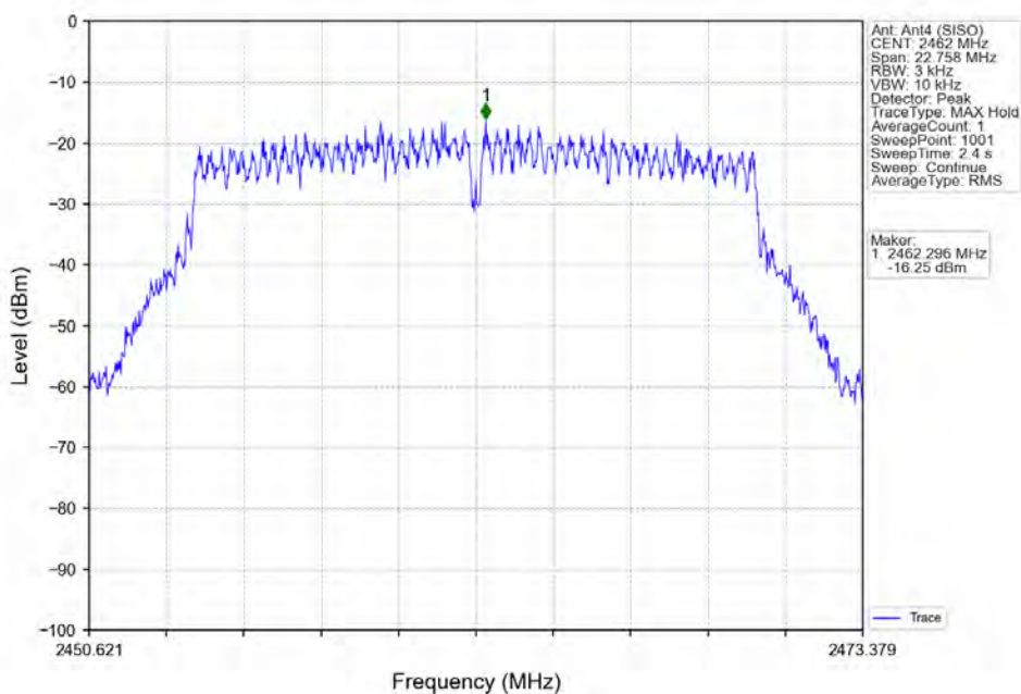
802.11g_HCH_2462MHz_Ant4 (SISO)_NTNV
