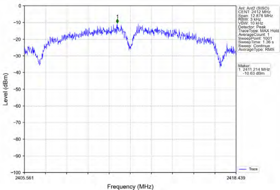
802.11b_LCH_2412MHz_Ant2 (SISO)_NTNV
