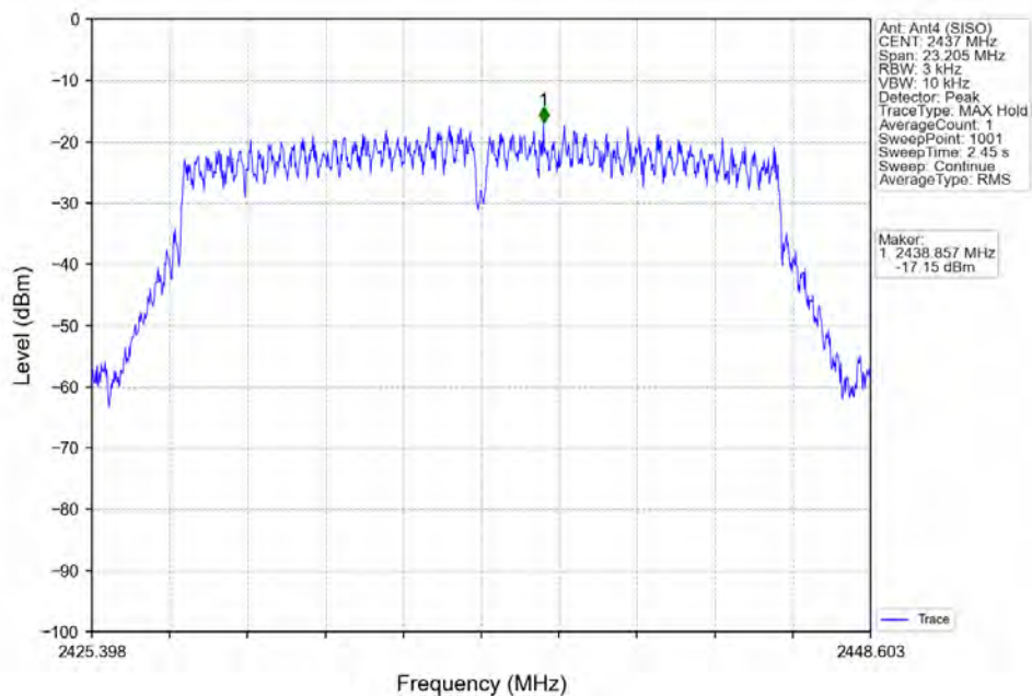
802.11n(HT20)_MCH_2437MHz_Ant4 (SISO)_NTNV
