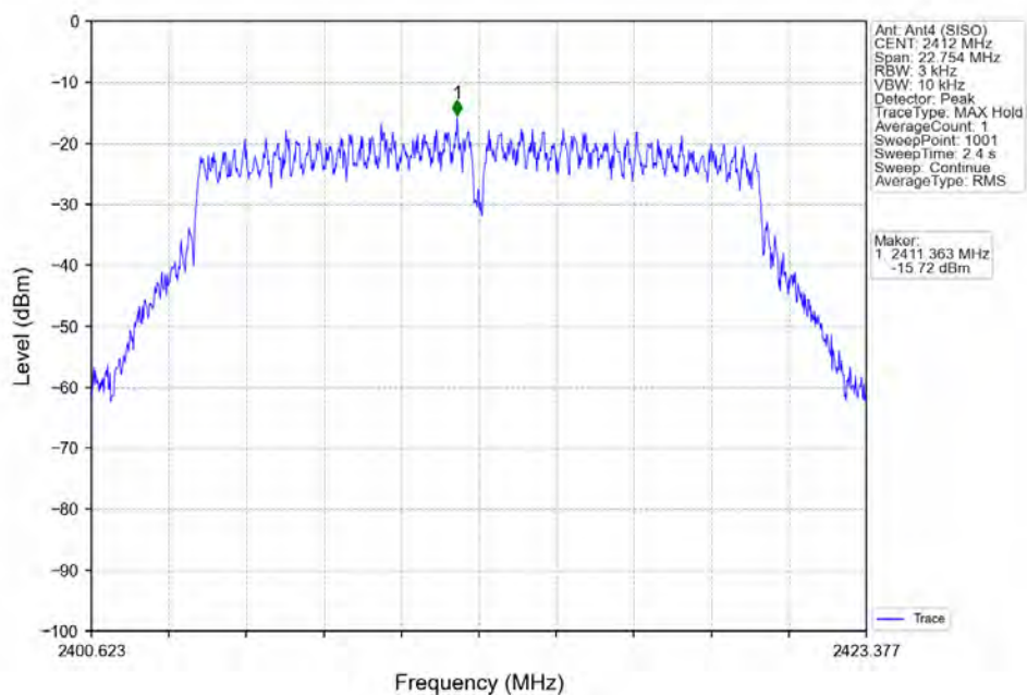
802.11g_LCH_2412MHz_Ant4 (SISO)_NTNV
