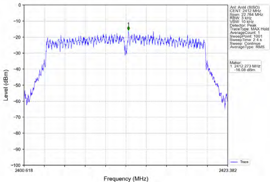
802.11n(HT20)_LCH_2412MHz_Ant4 (SISO)_NTNV
