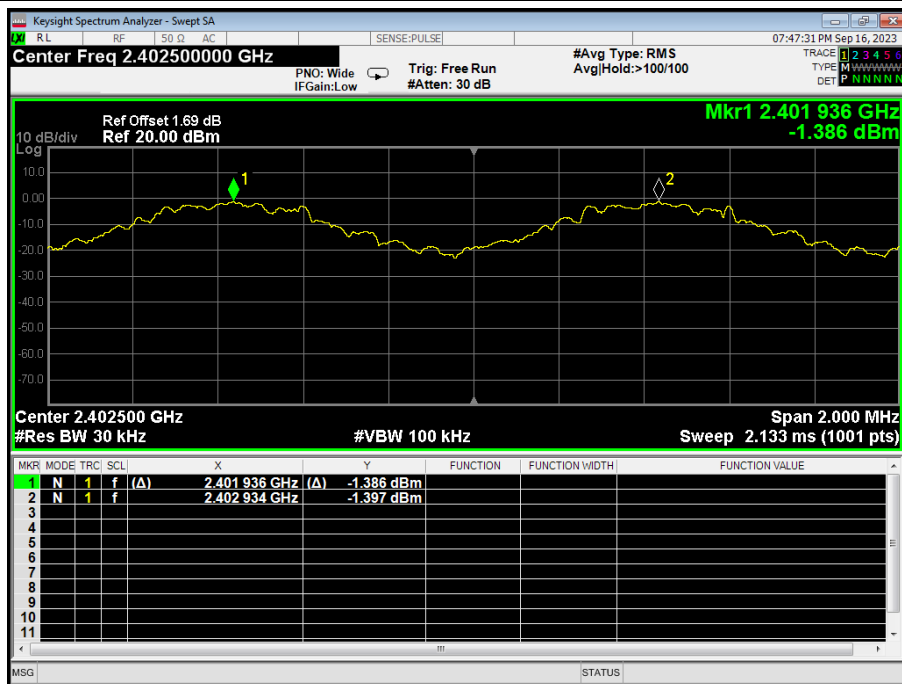
GFSK mode-CH00
