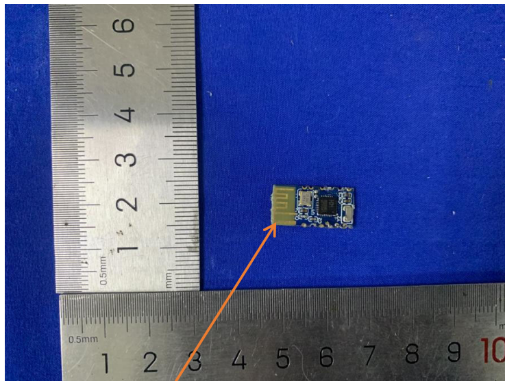
Antenna
