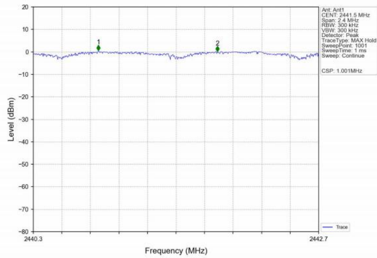
8DPSK_3DH5_HOPP_Ant1_NTNV
