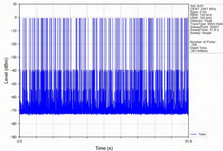
GFSK_DH3_HOPP_Ant1_NTNV
