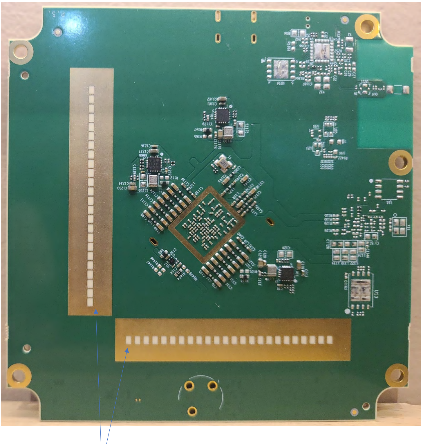
ANTENNA ARRAY
