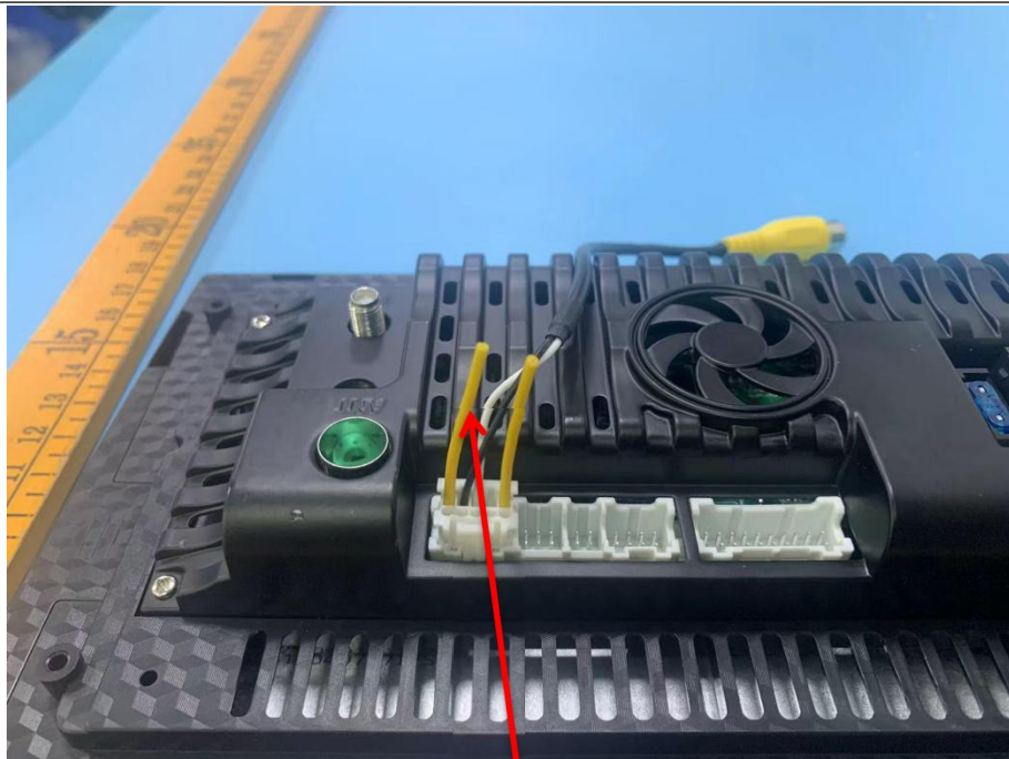
BT/WIFI--ANT
