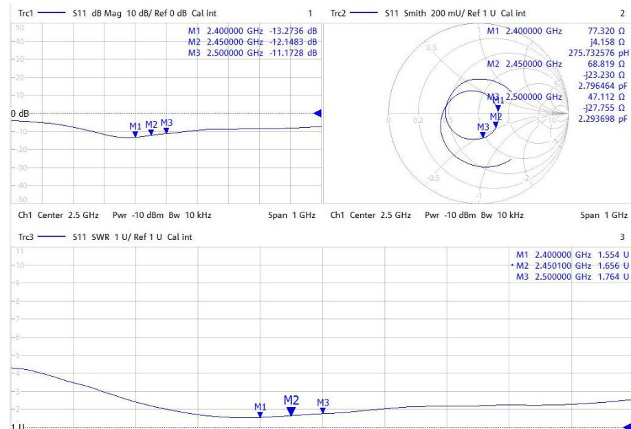
INPUT-ANT1 Electrical Performance Test Parameter Table
