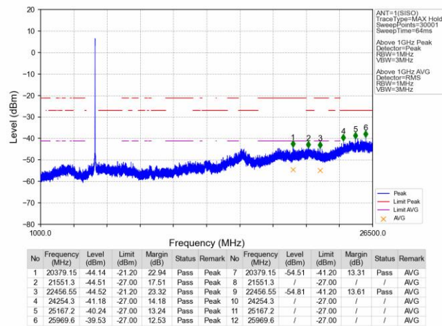
802.11a LCH 5180MHz_Ant1_NTNV
