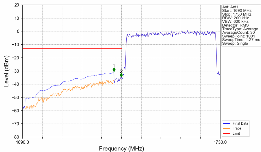
Band4_20MHz_QPSK_LCH_1720MHz_RB_100_0_NTNV
