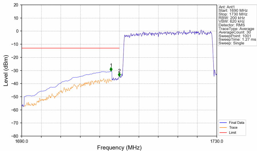
Band4_20MHz_16QAM_LCH_1720MHz_RB_100_0_NTNV
