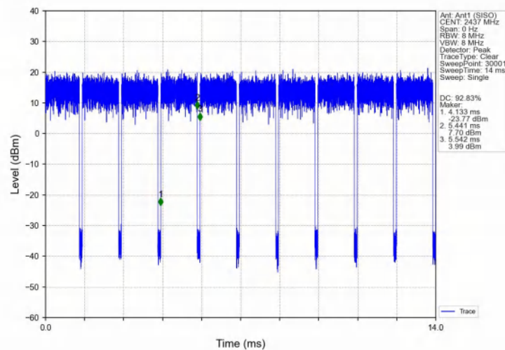
802.11n(HT20) MCH 2437MHz Ant1 (SISO) NTN
