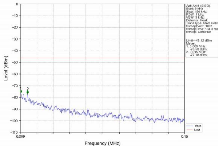
802.11n(HT20) LCH_2412MHz_Ant1 (SISO) NTV
