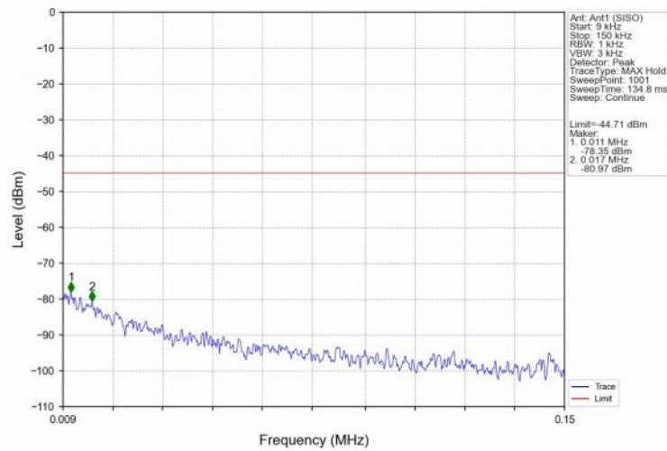
802.11b_HCH_2462MHz_Ant1 (SISO) NTN
