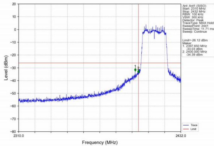
802.11n(HT20) LCH_2412MHz_Ant1 (SISO) NTV
