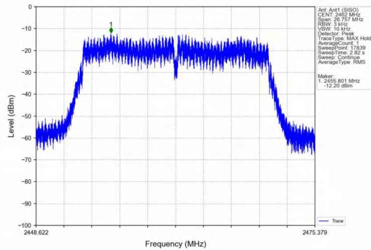
802.11n(HT20) HCH 2462MHz Ant1 (SISO) NTN
