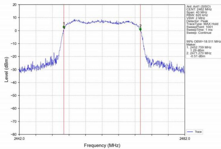
802.11n(HT20) HCH 2462MHz Ant1 (SISO) NTVN
