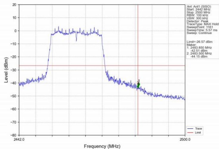
802.11n(HT20) HCH 2462MHz Ant1 (SISO) NTVN
