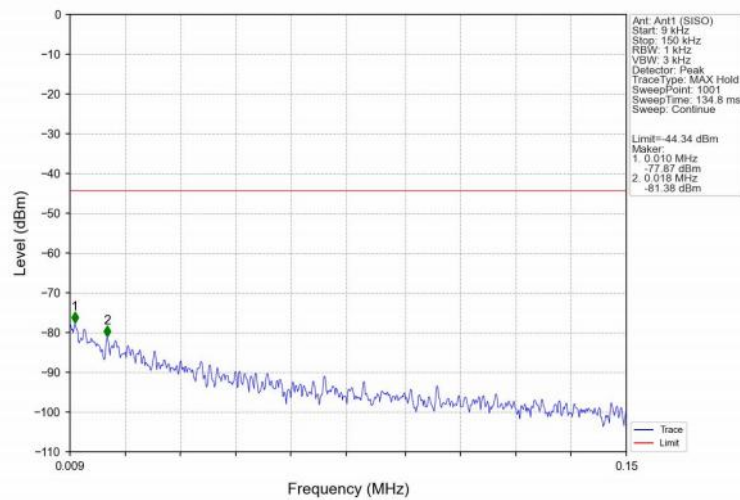
802.11b LCH 2412MHz Ant1 (SISO) NTN
