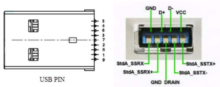
Figure 3 DAT interface pin diagram
