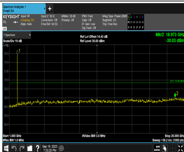
Band25-20MHz-16QAM-26365-1RB#0-Range2:1000~20000MHz
