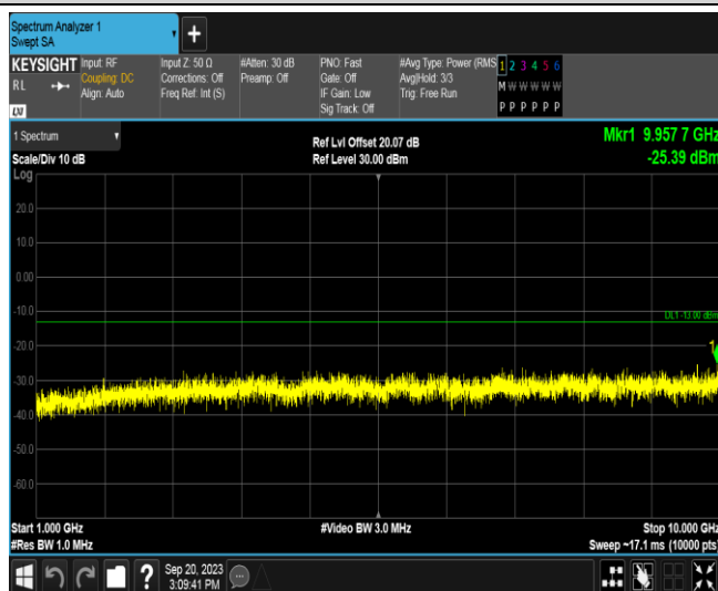
Band26A-5MHz-QPSK-26915-1RB#0-Range2:1000~10000MHz
