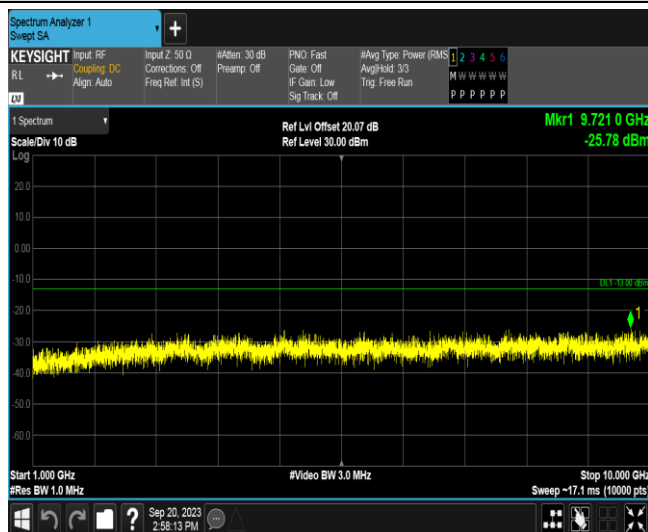
Band26A-3MHz-QPSK-27025-1RB#0-Range2:1000~10000MHz
