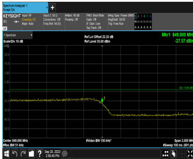
Band26A-3MHz-QPSK-27025-1RB#14
