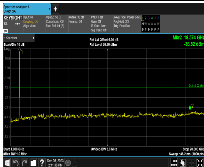
Band25-10MHz-QPSK-26365-1RB#0-Range2:1000~20000MHz
