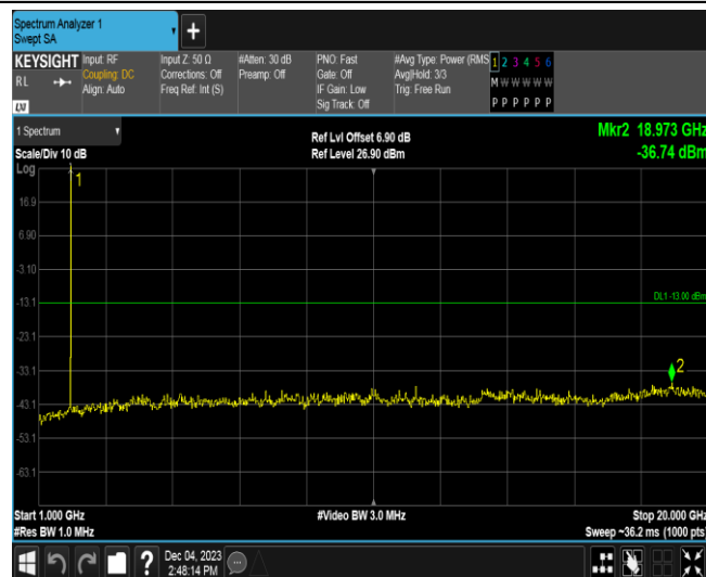
Band2-5MHz-QPSK-19175-1RB#0-Range2:1000~20000MHz
