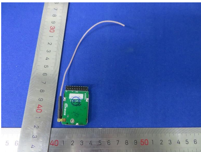
Antenna 3# :
