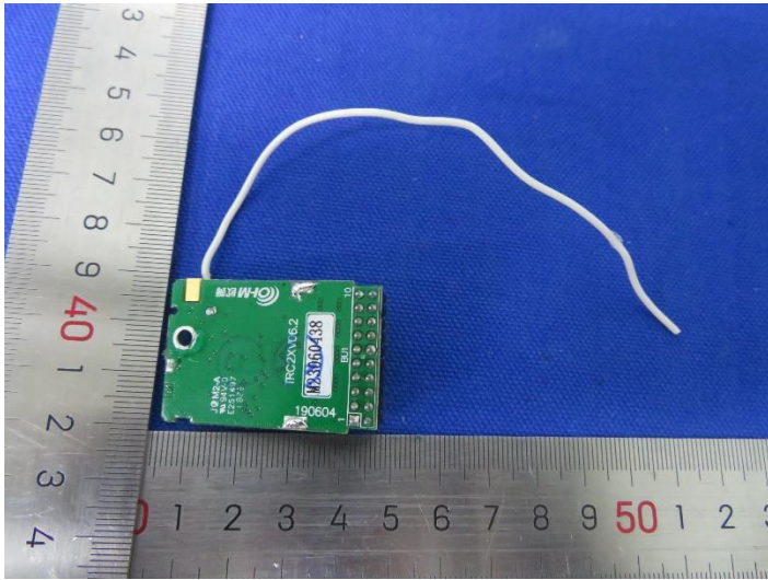
Antenna 2# :
