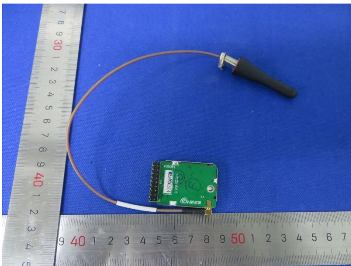
Antenna 3# :
