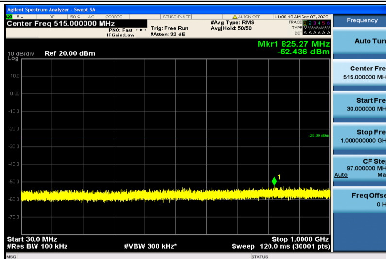
Band7-20MHz-QPSK-21350-1RB#0-30~1000MHz
