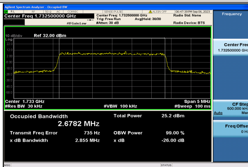
Band4-3MHz-QPSK-17325-15RB#0-2.6782
