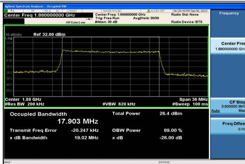
Band2-20MHz-QPSK-18900-100RB#0-17.903
