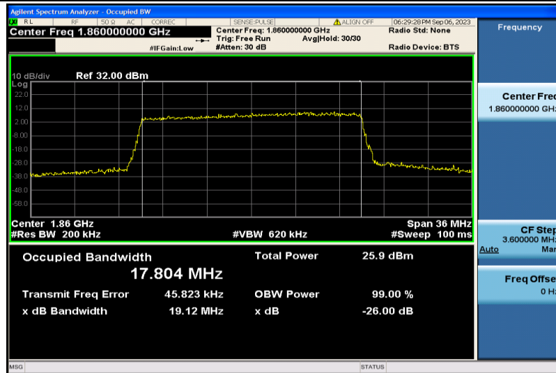
Band2-20MHz-QPSK-18700-100RB#0-17.804
