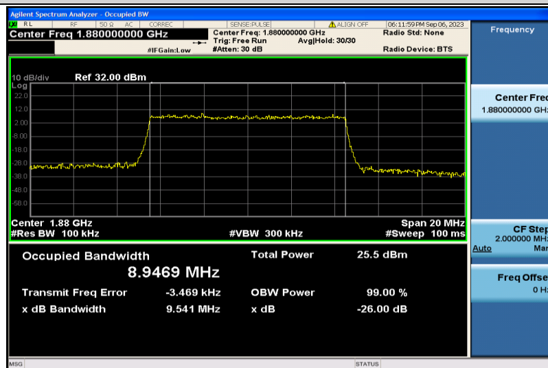
Band2-10MHz-QPSK-18900-50RB#0-8.9469
