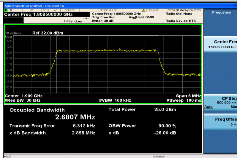
Band2-3MHz-QPSK-19185-15RB#0-2.6807
