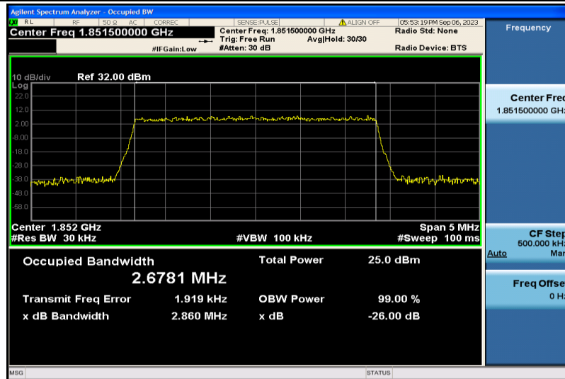
Band2-3MHz-QPSK-18615-15RB#0-2.6781
