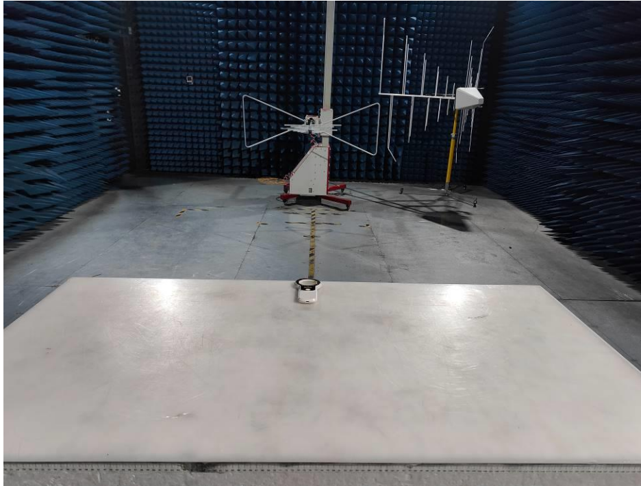
30MHz-1000MHz
