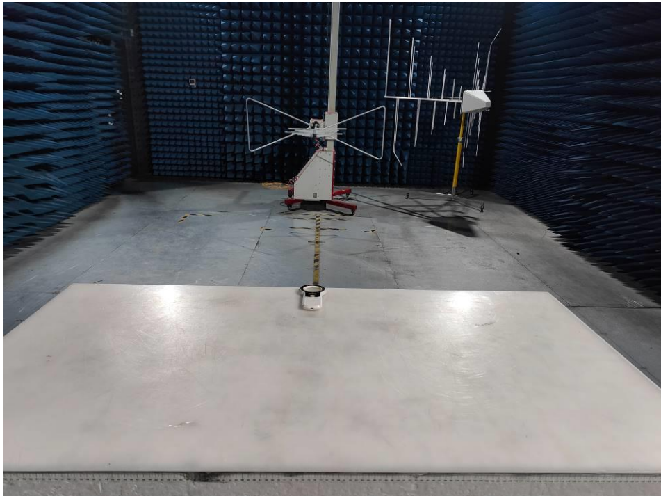
30MHz-1000MHz
