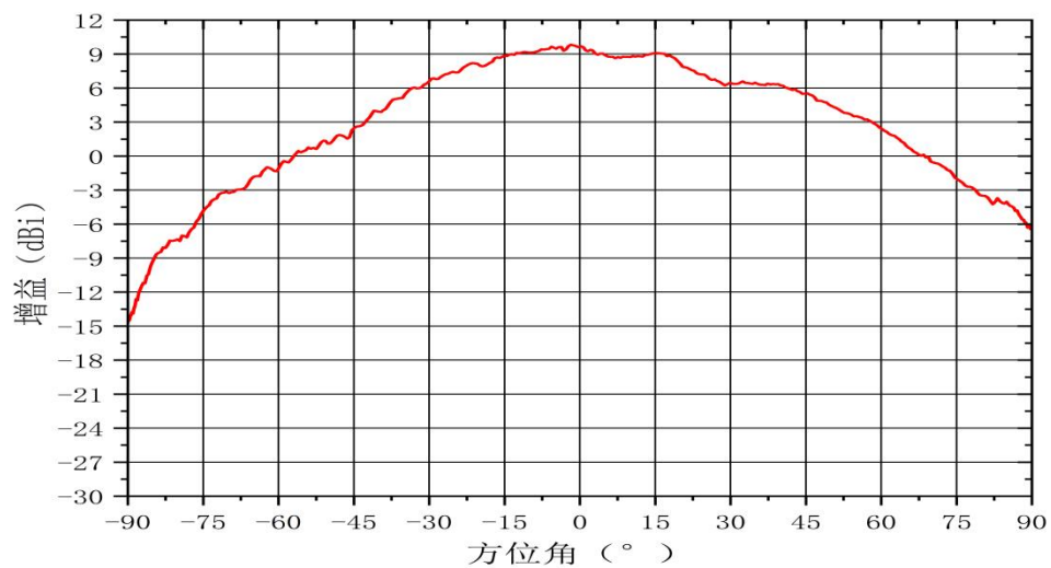
方位面方向图(TX0) Freq:59.0GHz
