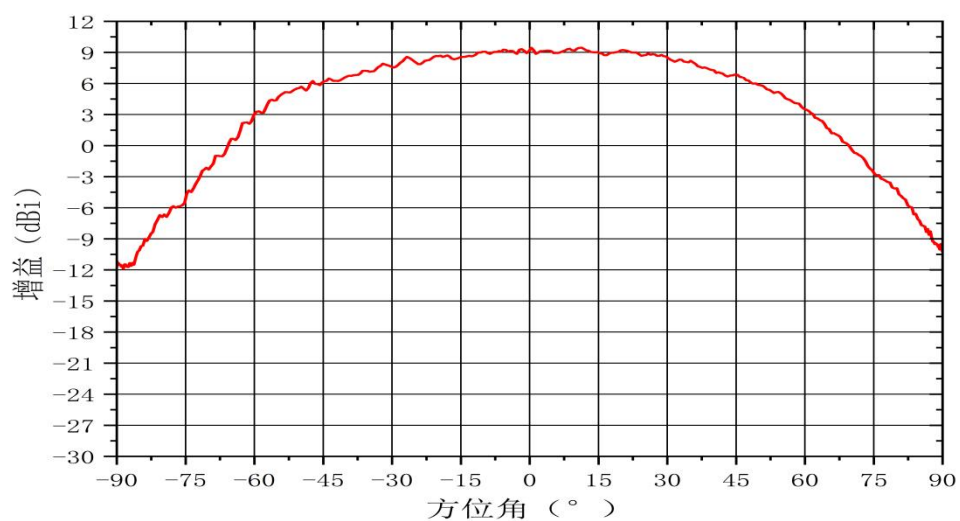
方位面方向图(TX1)Freq:58.0GHz
