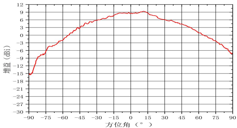
方位面方向图(TX0) Freq:58.0GHz
