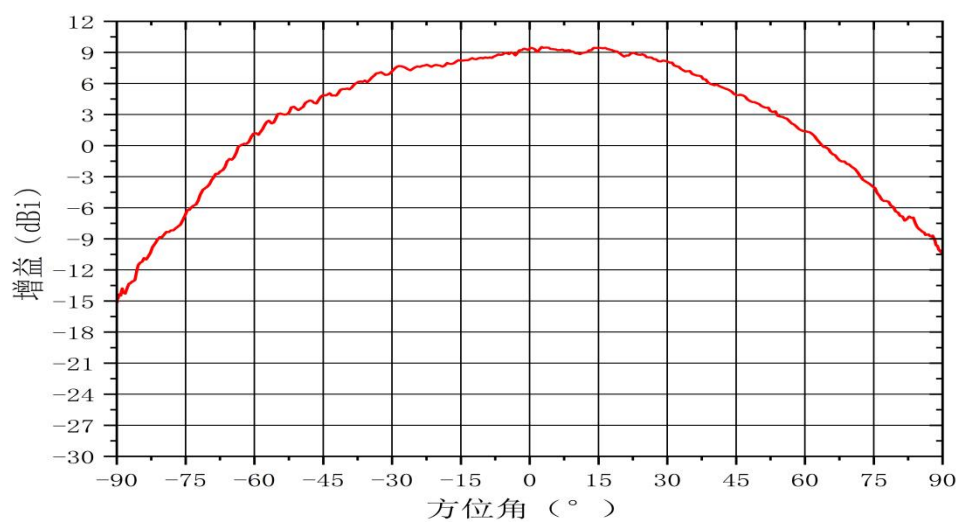
方位面方向图(TX1)Freq:59.0GHz
