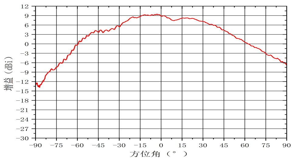
方位面方向图(TX0)Freq:61.0GHz
