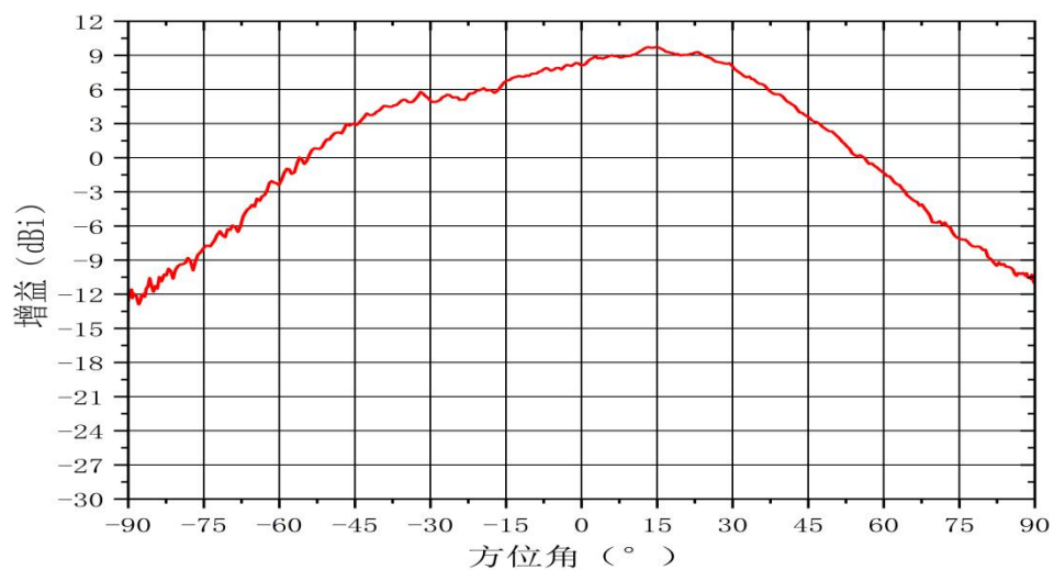
方位面方向图(TX1)Freq:61.0GHz
