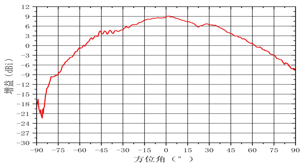
方位面方向图(TX0) Freq:57.0GHz
