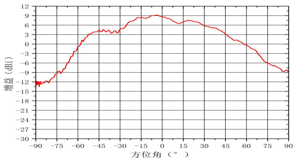
方位面方向图(TX0)Freq:62.0GHz
