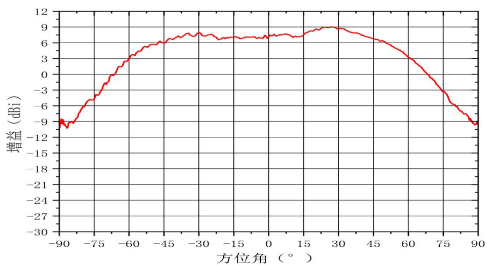
方位面方向图(TX1)Freq:57.0GHz
