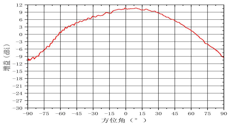
方位面方向图(TX1)Freq:60.0GHz
