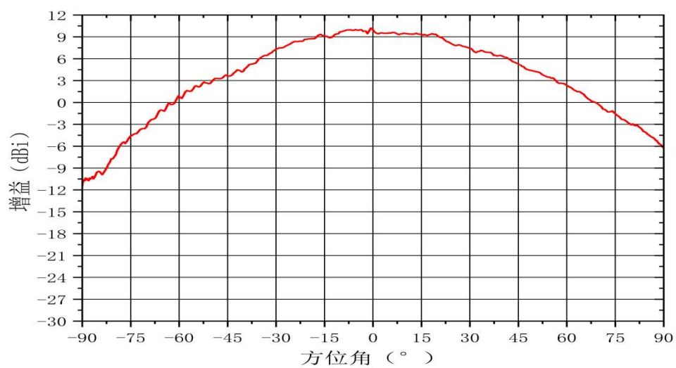
方位面方向图(TX0)Freq:60.0GHz
