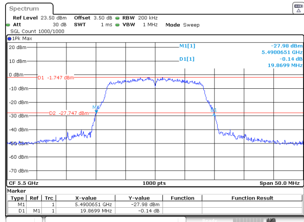
802.11a_5500MHz
