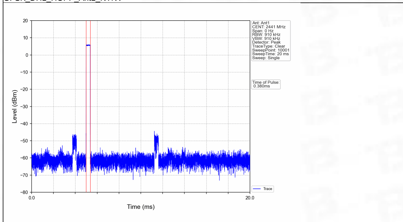
GFSK_DH1_HOPP_Ant1_NTNV
