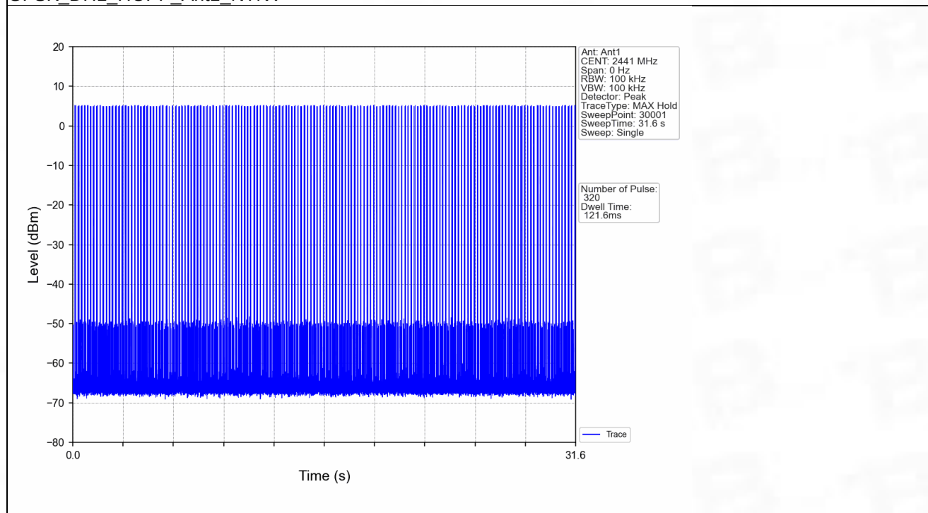
GFSK_DH1_HOPP_Ant1_NTNV
