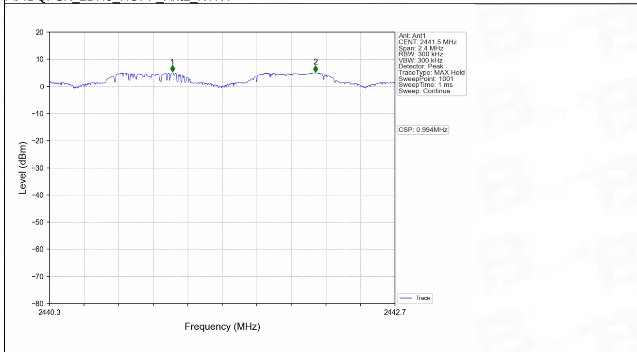
Pi/4DQPSK_2DH5_HOPP_Ant1_NTNV
