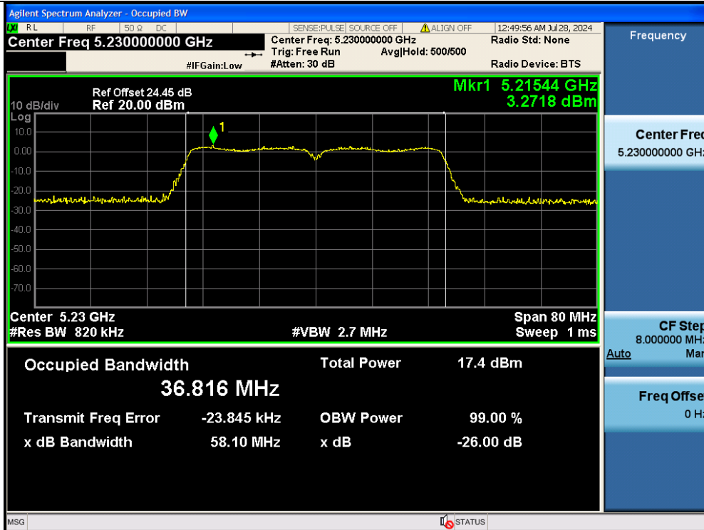
11N40MIMO-Ant2-5230
