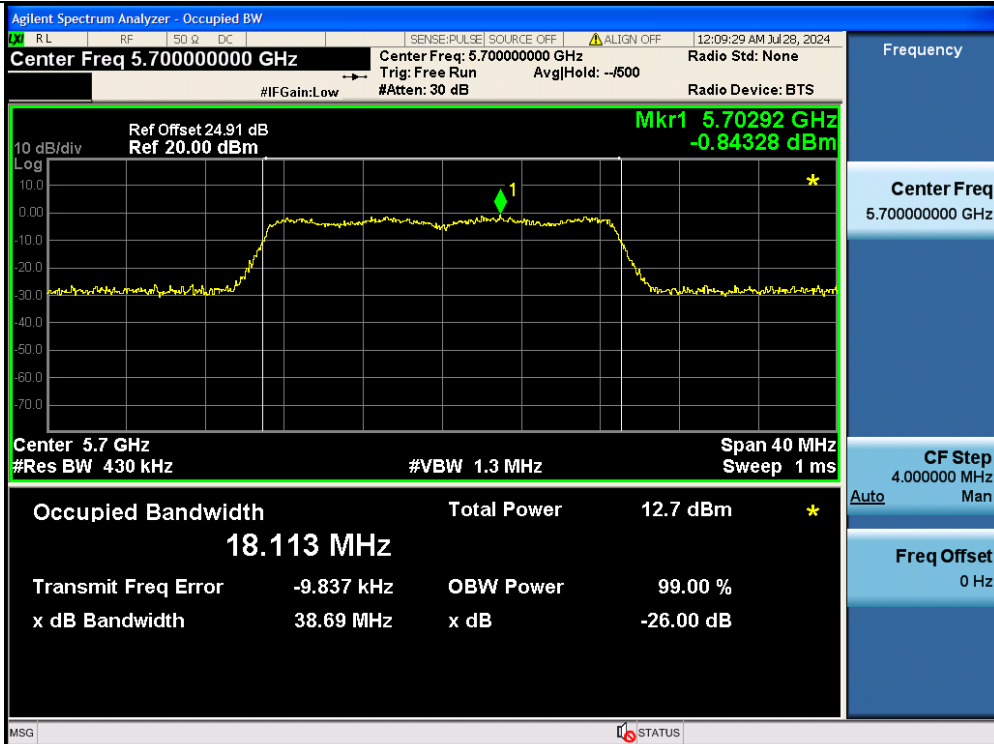
11N20MIMO-Ant2-5700
