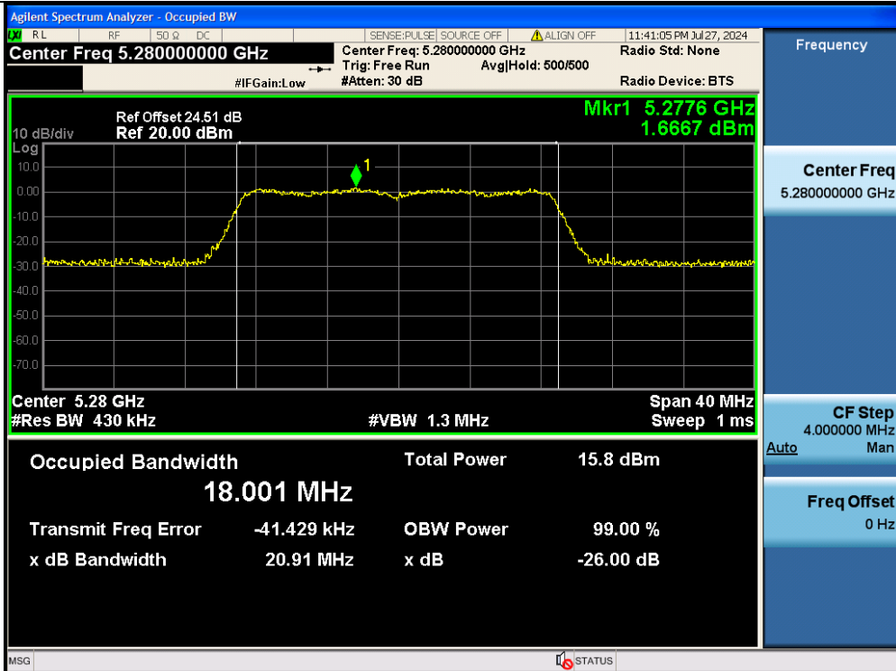
11N20MIMO-Ant2-5280
