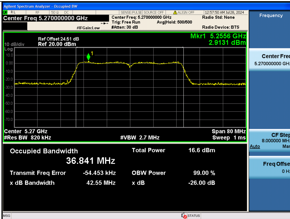
11N40MIMO-Ant2-5270
