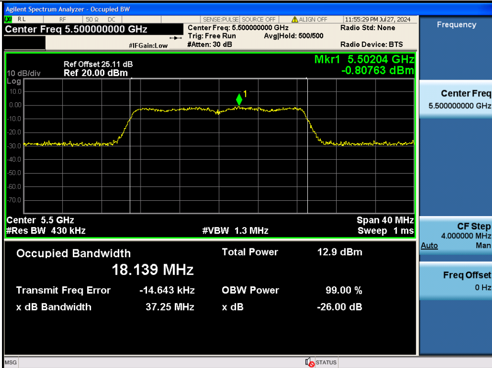
11N20MIMO-Ant2-5500
