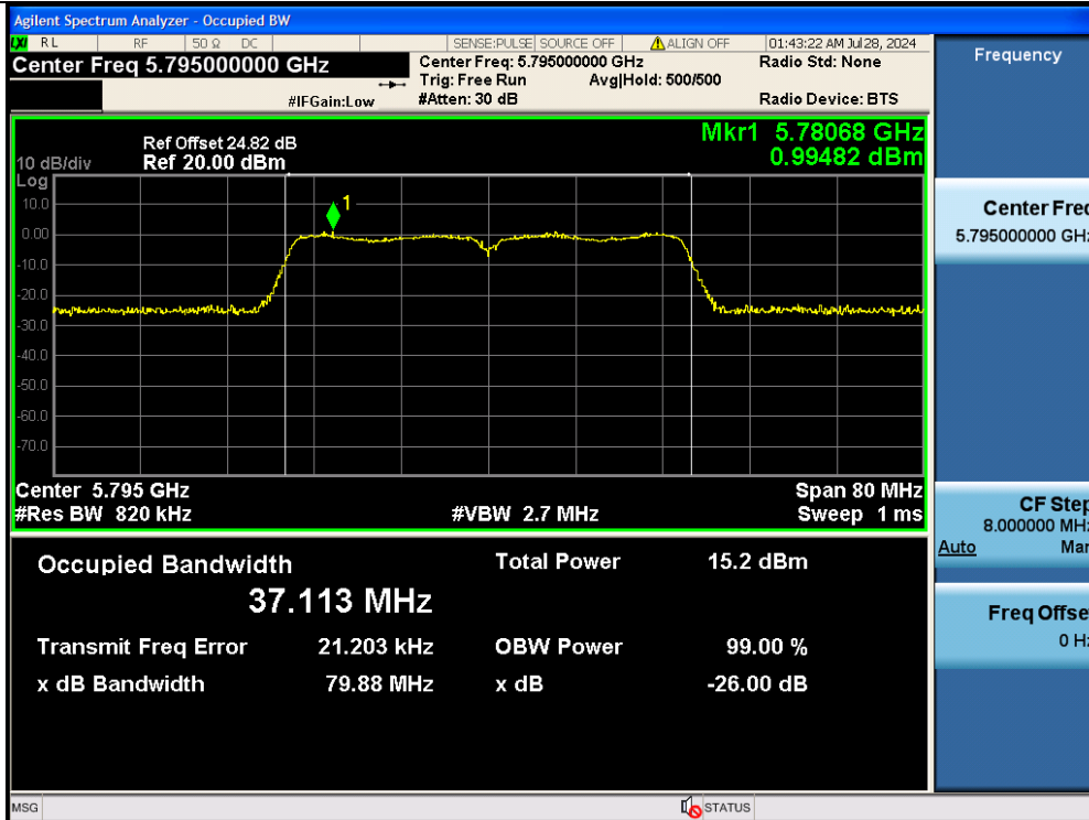
11N40MIMO-Ant2-5795
