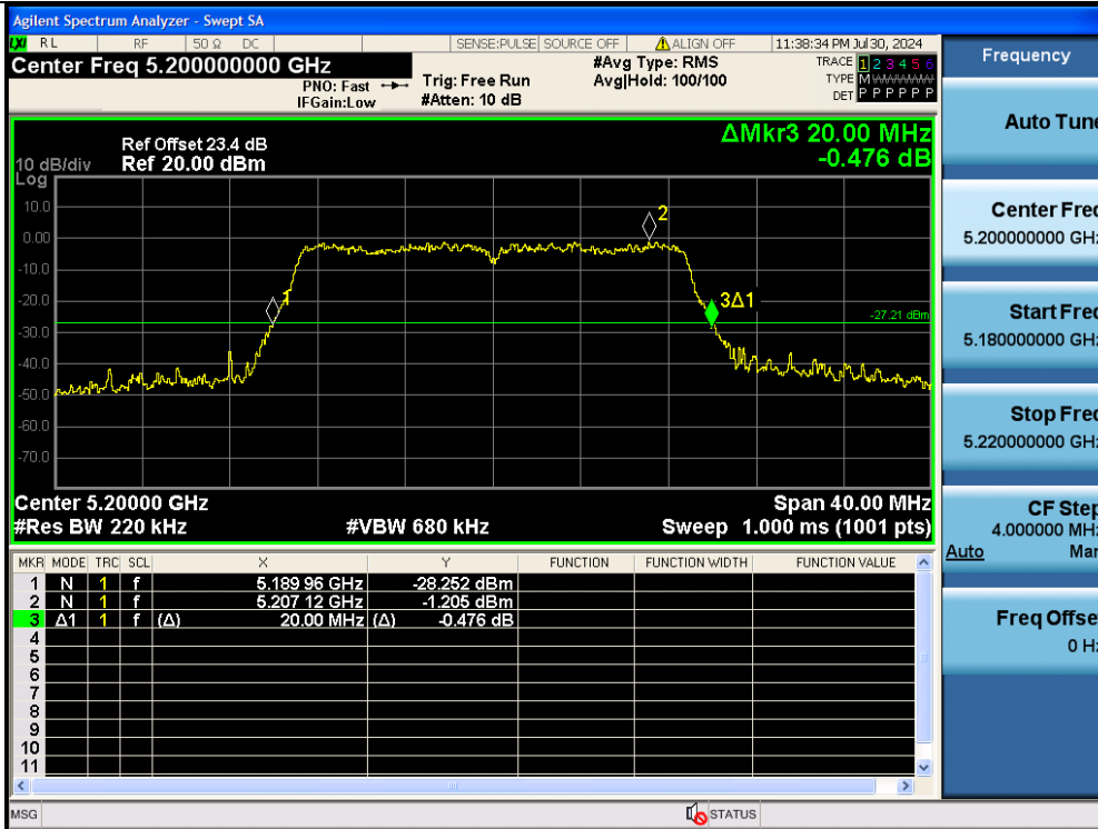
11N20MIMO-Ant2-5200
