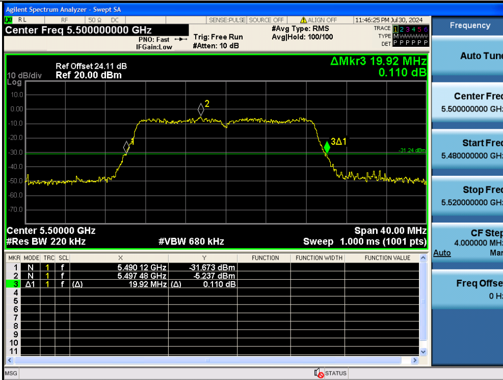
11N20MIMO-Ant2-5500
