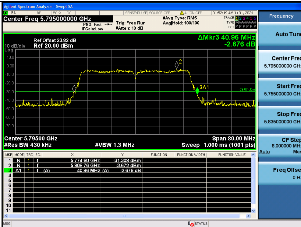
11N40MIMO-Ant2-5795
