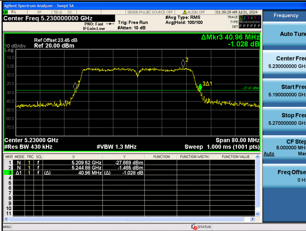
11N40MIMO-Ant2-5230
