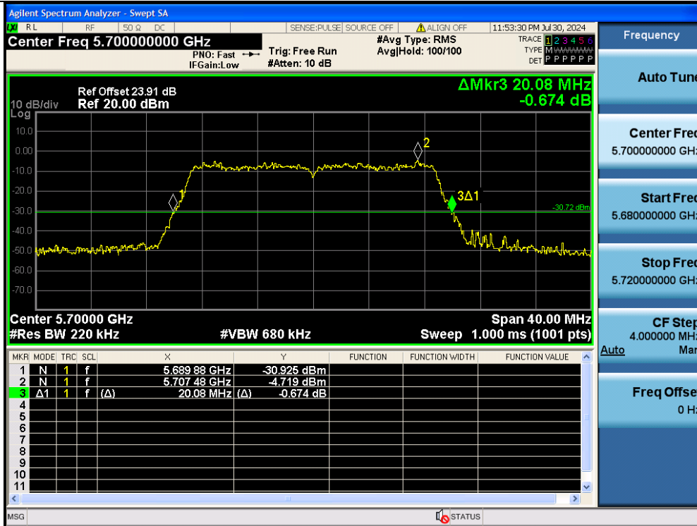
11N20MIMO-Ant2-5700
