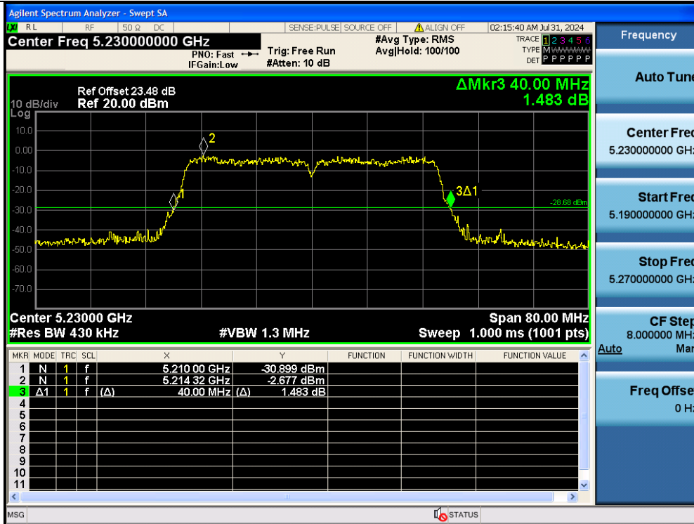
11AC40MIMO-Ant1-5230
