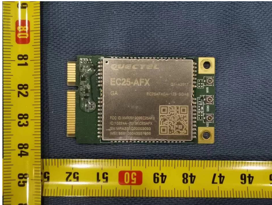
EUT Photo(LTE module FCC ID: XMR201909EC25AFX, IC:10224A-2019EC25AFX)
