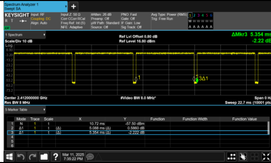
IEEE 802.11n_20MHz_Channel 1
