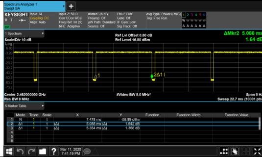
IEEE 802.11n_20MHz_Channel 11
