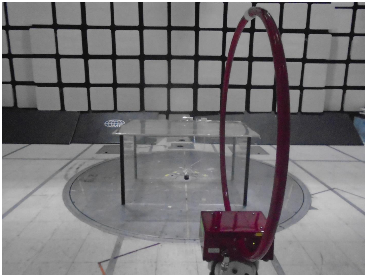
9kHz – 30MHz (Antenna View)
