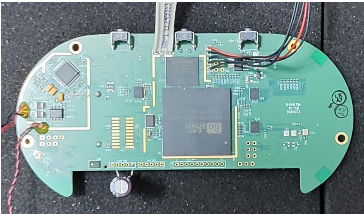
Hälsa Hub PCB Bottom side
