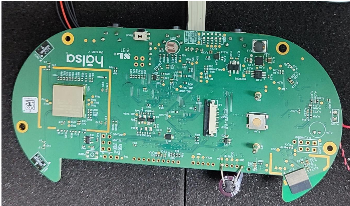
Hälsa Hub PCB Top side
