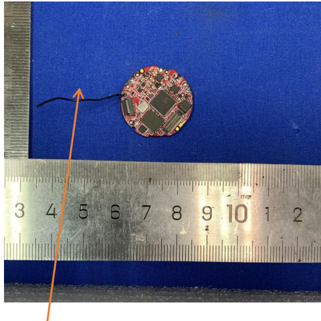
Antenna
