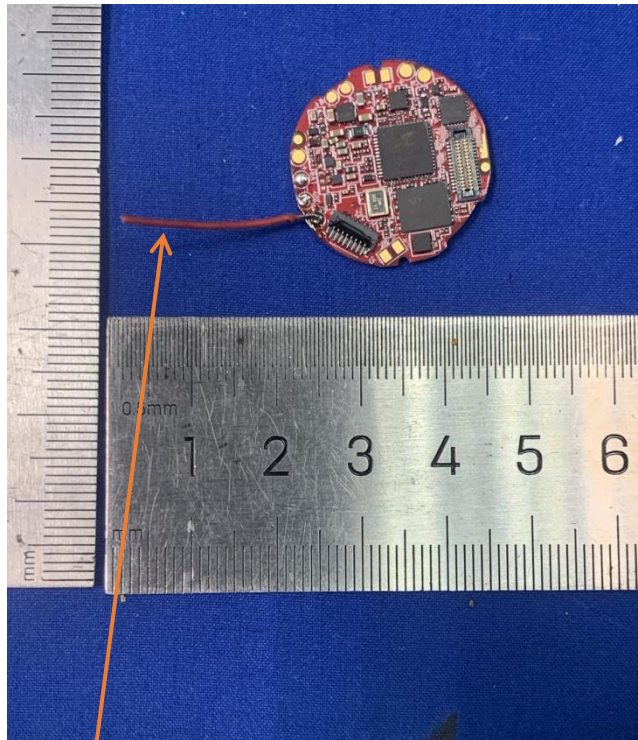
Antenna
