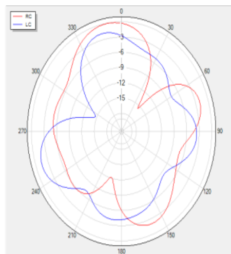
Theta=90 freq=2400MHz
