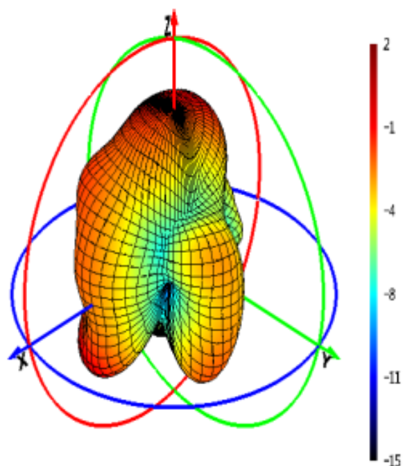
Theta=90 freq=2400MHz
