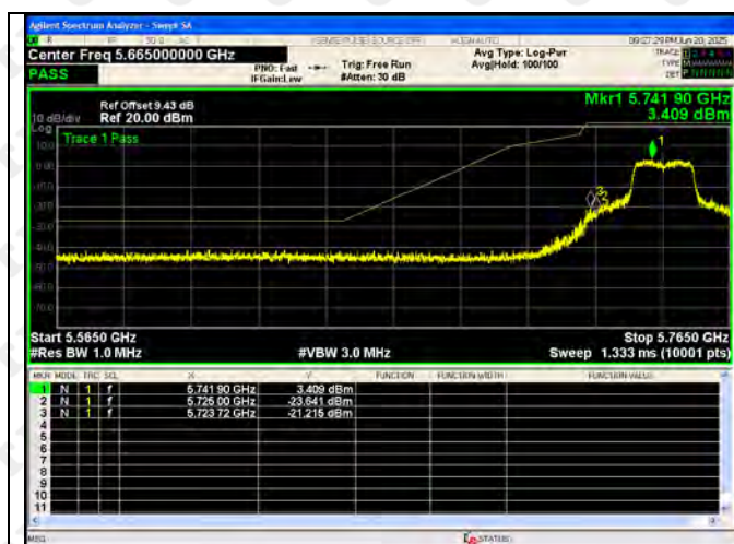
802.11(n40)-5755
