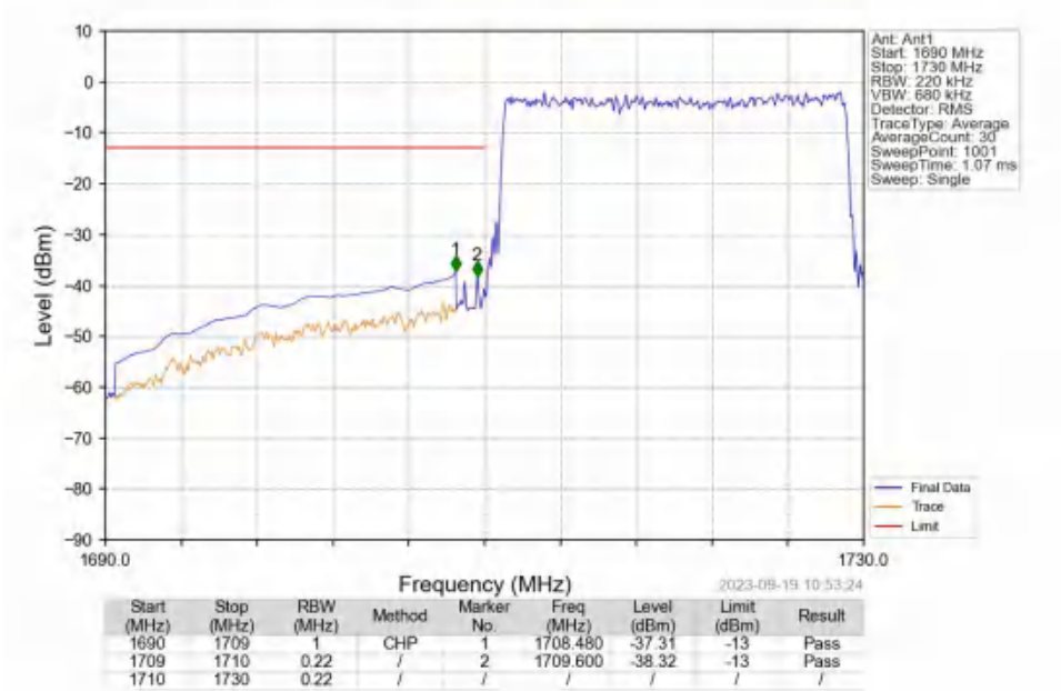
Band4_20MHz_QPSK_LCH_1720MHz_RB_100_0_NTNV
