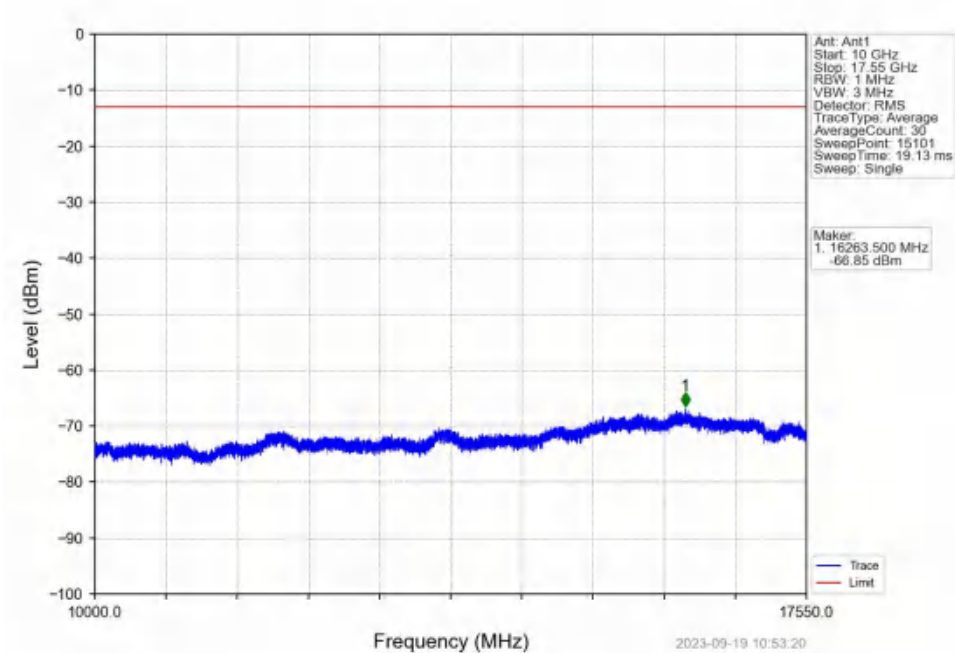
Band4_20MHz_QPSK_LCH_1720MHz_RB_1_0_NTNV
