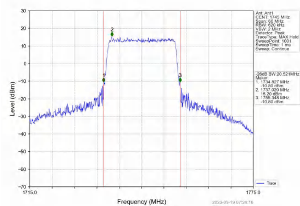
Band4_20MHz_QPSK_HCH_1745MHz_RB_100_0_NTNV
