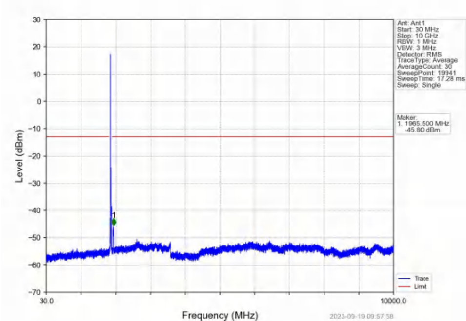
Band2_20MHz_QPSK_MCH_1880MHz_RB_1_0_NTNV
