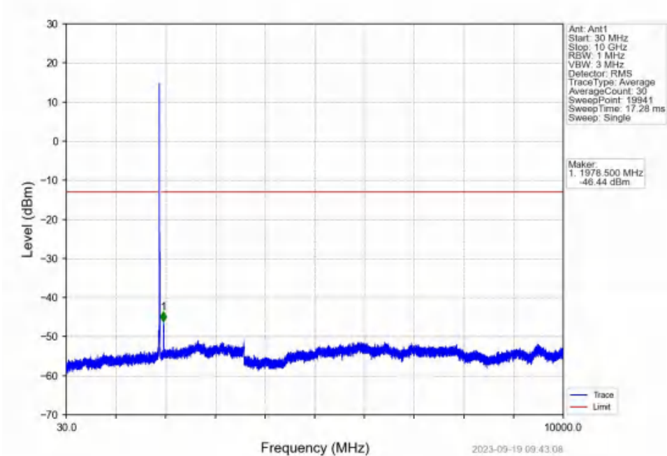
Band2_15MHz_QPSK_HCH_1902.5MHz_RB_1_0_NTNV
