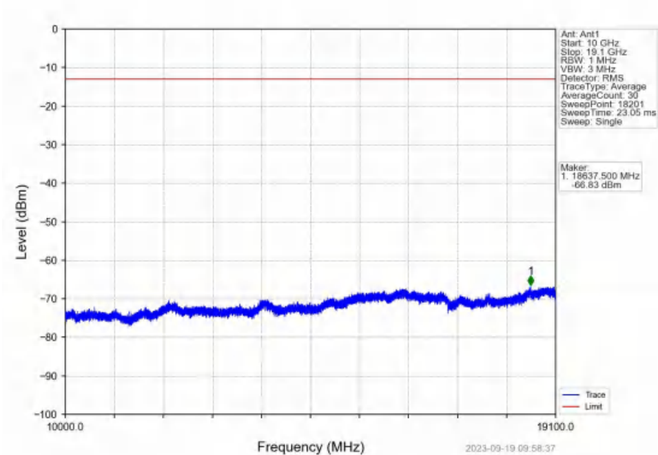
Band2_20MHz_QPSK_HCH_1900MHz_RB_1_0_NTNV
