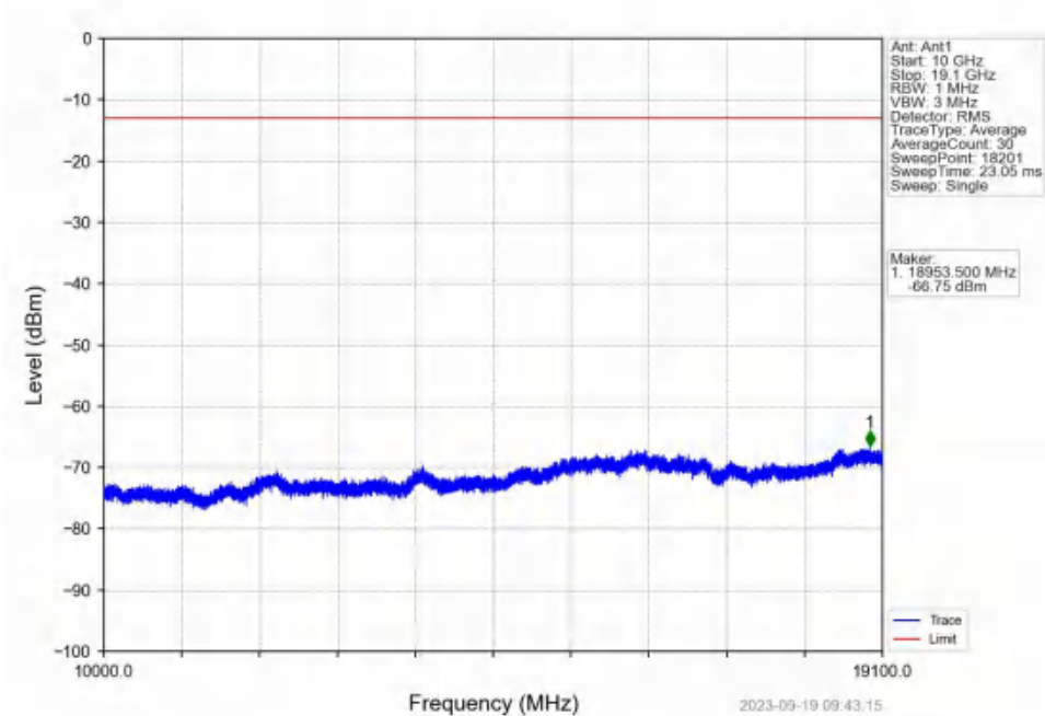
Band2_15MHz_QPSK_HCH_1902.5MHz_RB_1_0_NTNV
