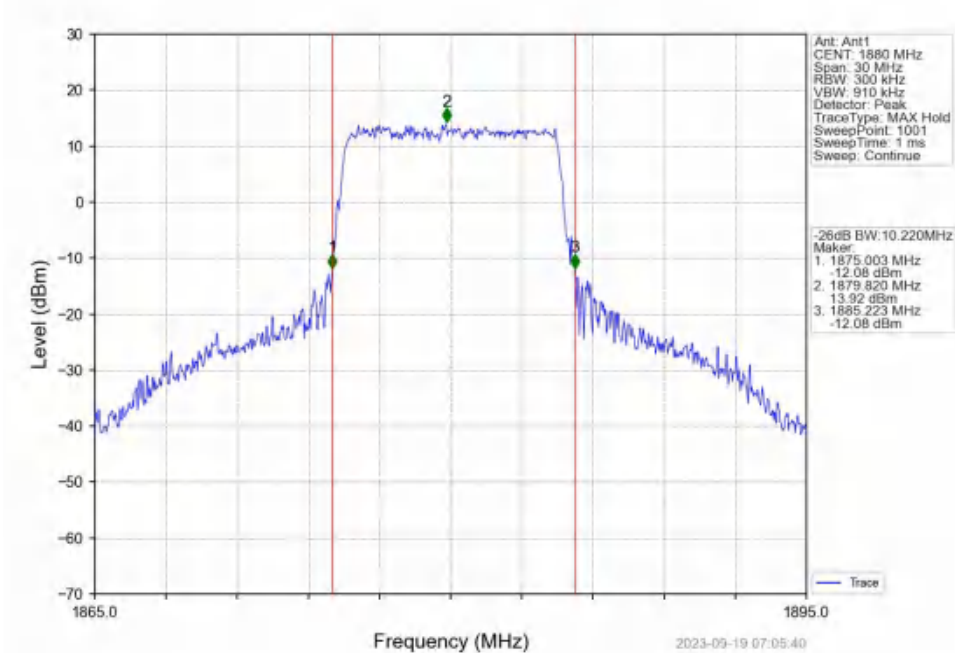
Band2_10MHz_16QAM_MCH_1880MHz_RB_50_0_NTNV
