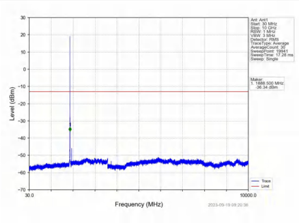
Band2_3MHz_16QAM_MCH_1880MHz_RB_1_0_NTNV
