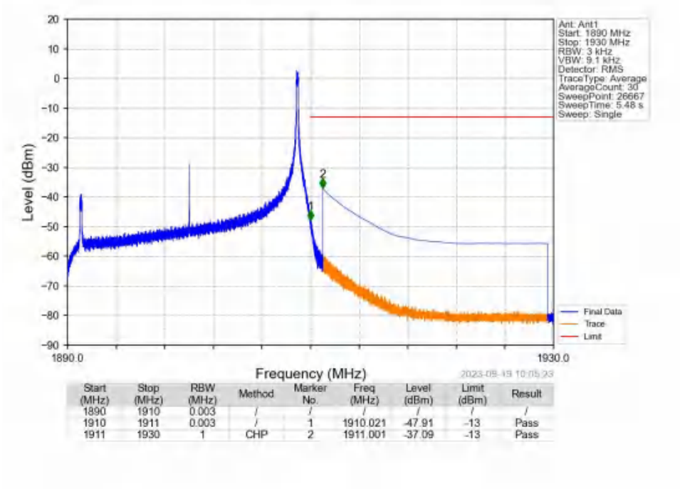
Band2_20MHz_16QAM_HCH_1900MHz_RB_100_0_NTNV
