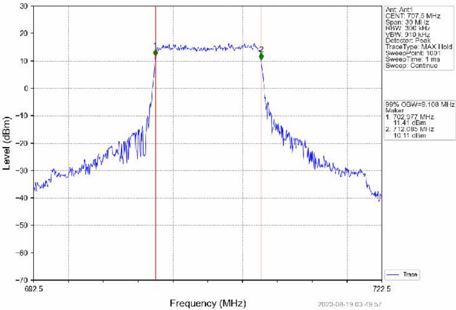
Band12_10MHz_QPSK_MCH_707.5MHz_RB_50_0_NTNV
