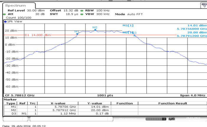
SRD 1.4MHz CA_Ant1_5788.12
