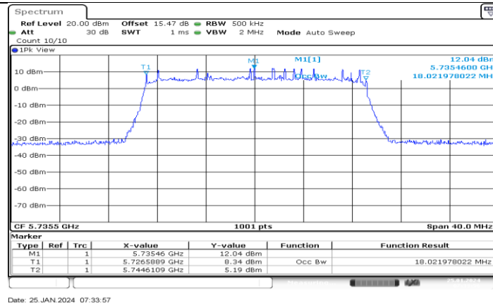
SRD 20MHz_Ant1_5735.5
