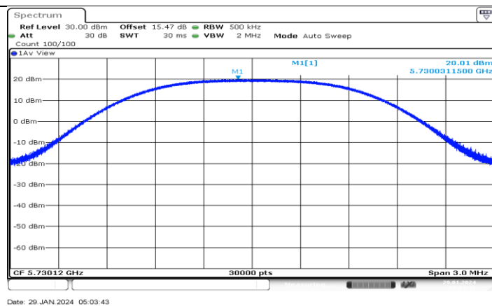
SRD 1.4MHz CA_Ant1_5730.12
