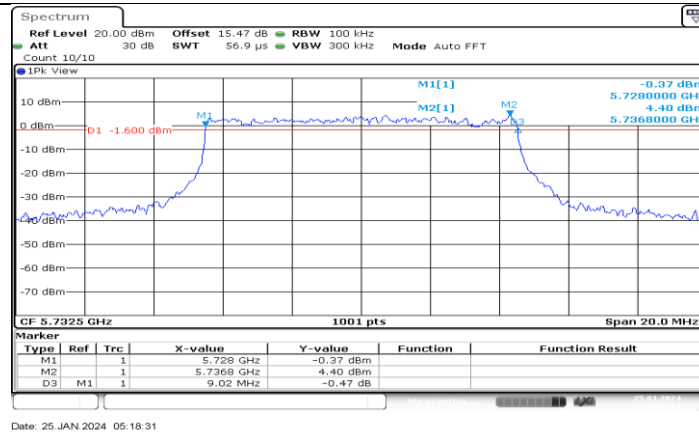
SRD 10MHz_Ant1_5732.5
