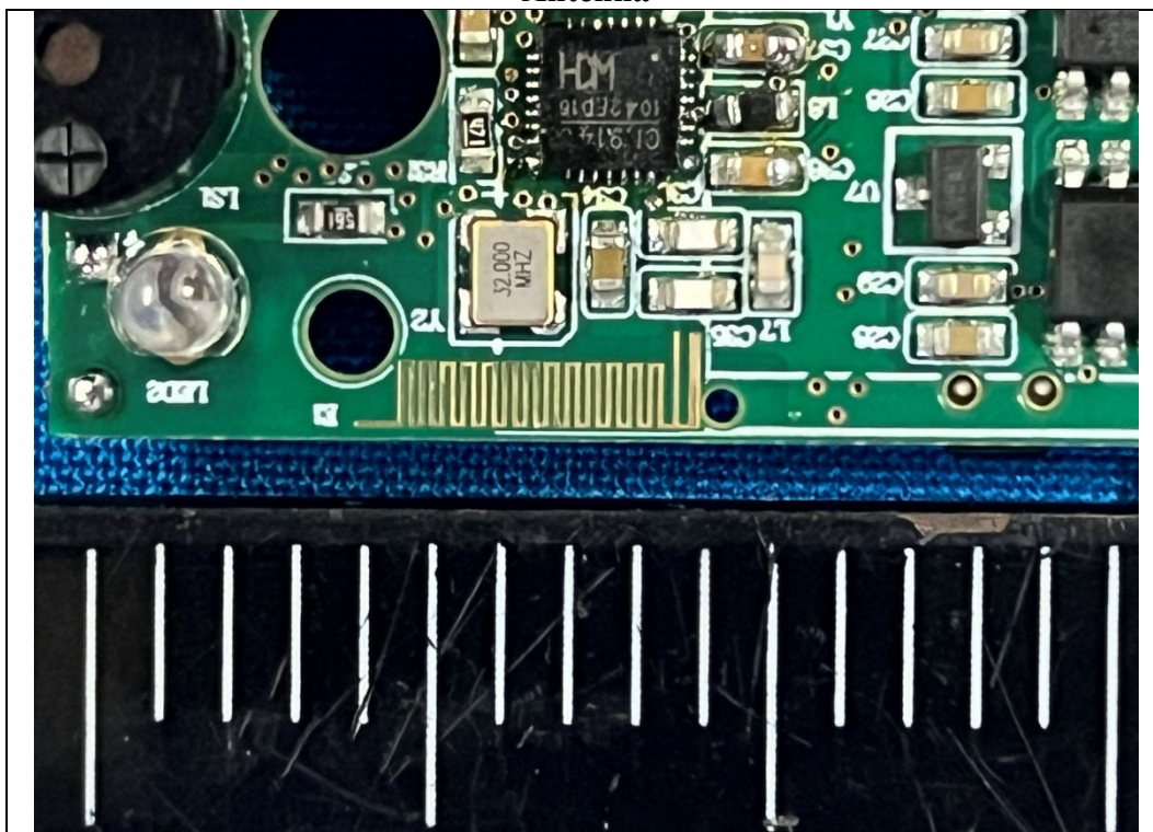
Module-CH9143
