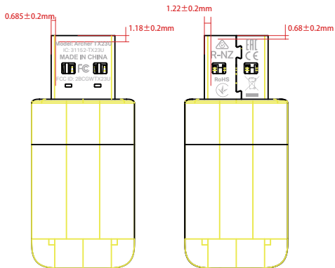
尺寸图
