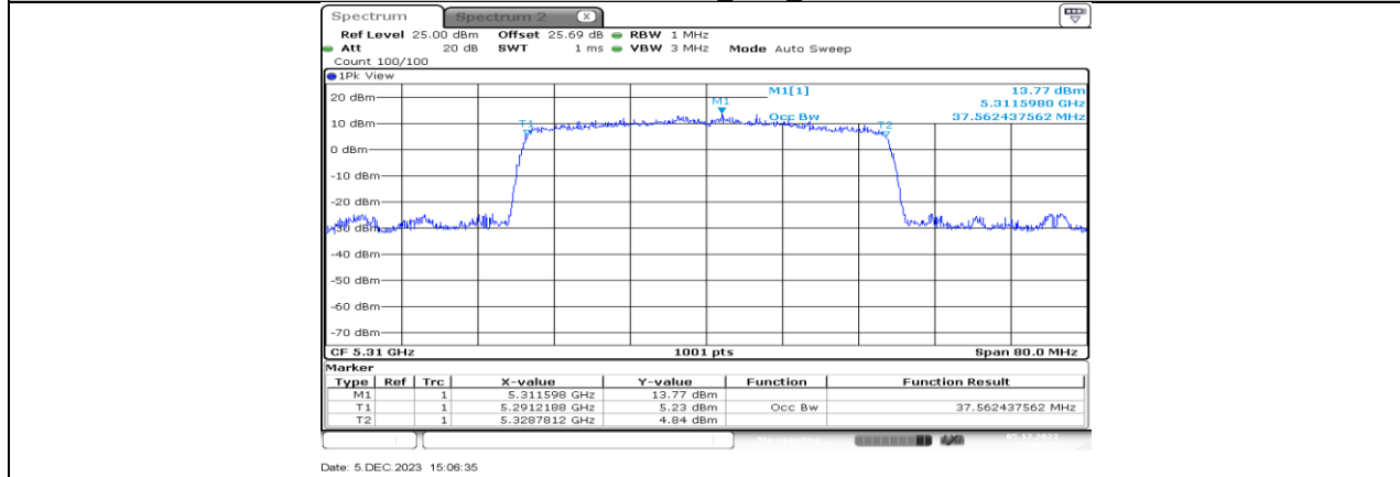
11AX40MIMO_Ant1_5310
