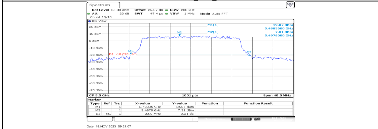
11AX20MIMO_Ant2_5500
