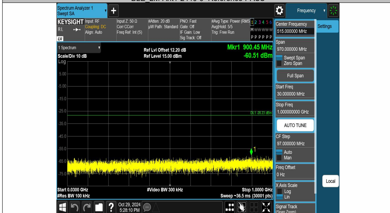
BLE_2M-Ant1-2440-30~1000-PASS
